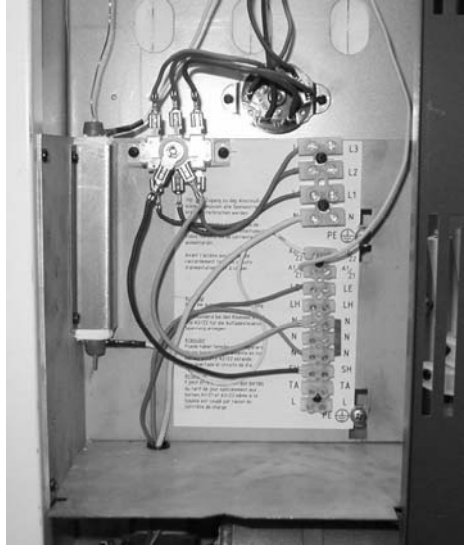
Fig.1 Thermisches Freigabeschütz
