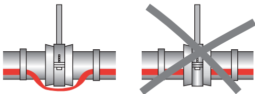
Abbildung 3: Band über Rohraufhängungen führen, Band nicht klemmen!
