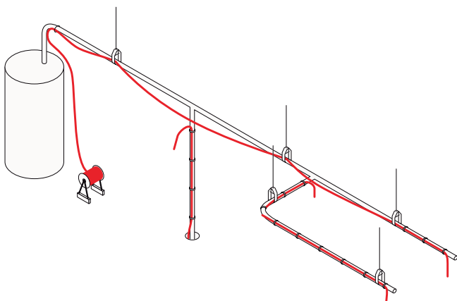
Abbildung 4: Auslegung des HWAT-Bands
