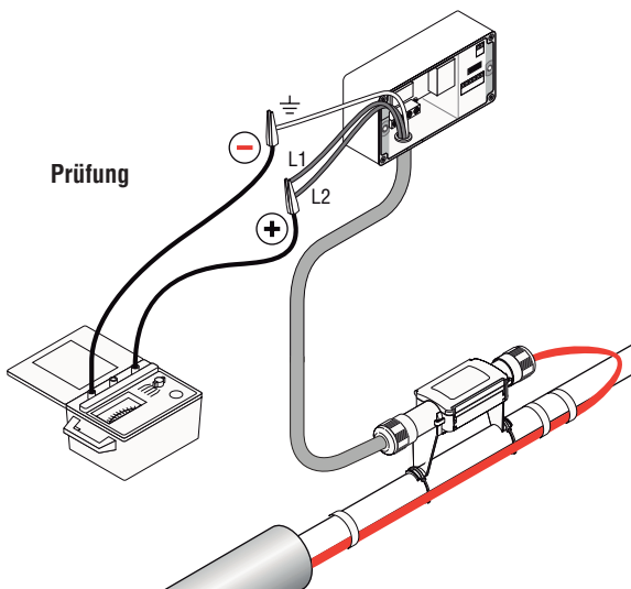
Abbildung 10: Isolationswiderstandsprüfung
