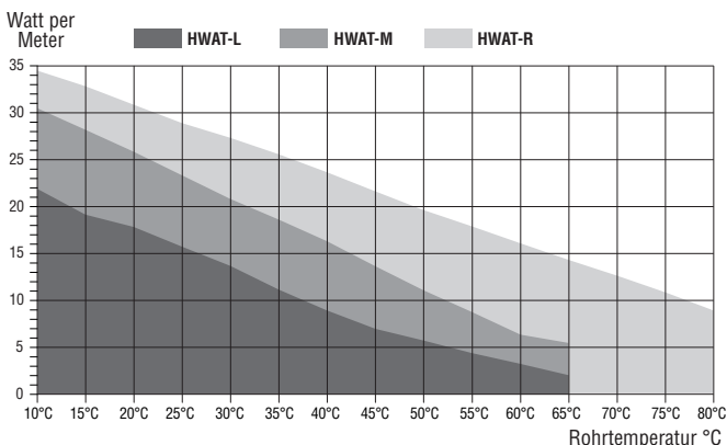
Abbildung 3: Leistungsabgabe bei AC 230 V auf gedämmten Stahlrohren
