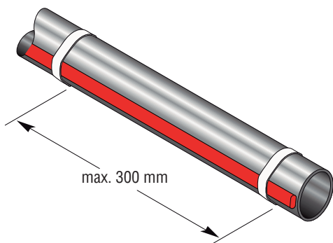
Abbildung 7: Befestigen des Temperaturhaltebands
