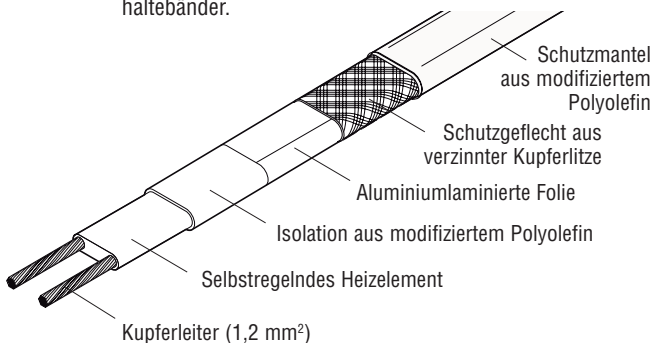
Abbildung 2: Temperaturhaltebänder HWAT-L, HWAT-M und HWAT-R
